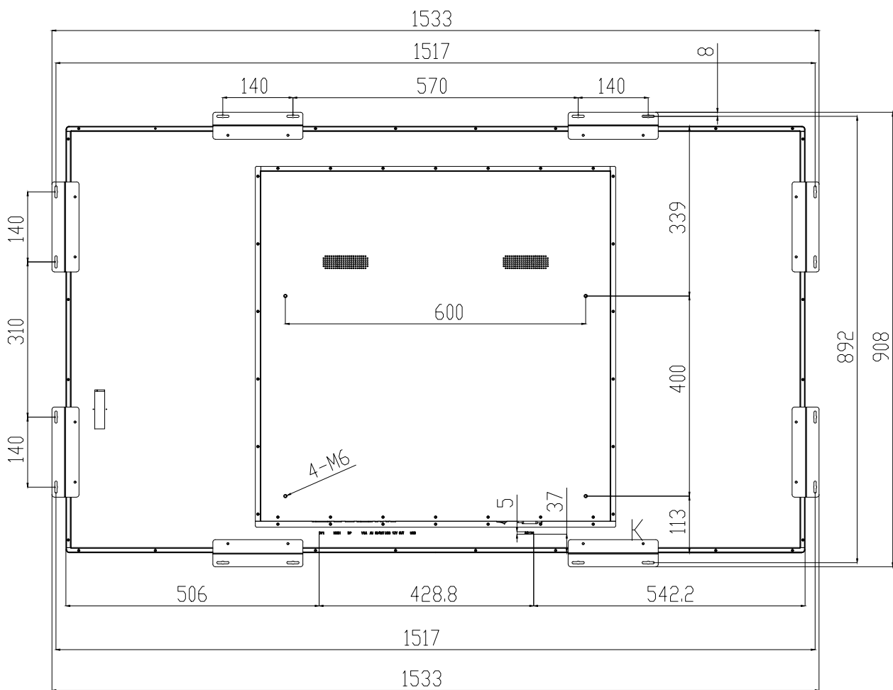
СХЕМА ДИСПЛЕЯ (ВИД СЗАДИ)
