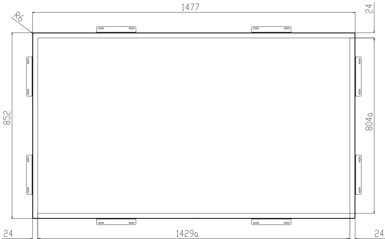
СХЕМА ДИСПЛЕЯ (ВИД СПЕРЕДИ)
