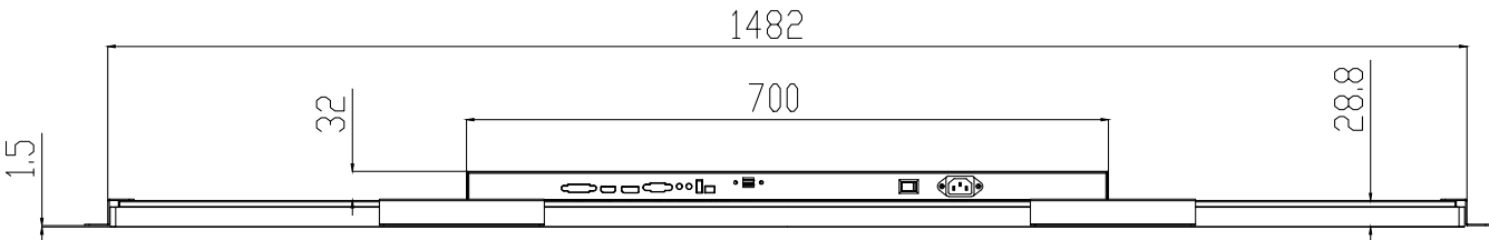
СХЕМА ДИСПЛЕЯ (ВИД СНИЗУ)
